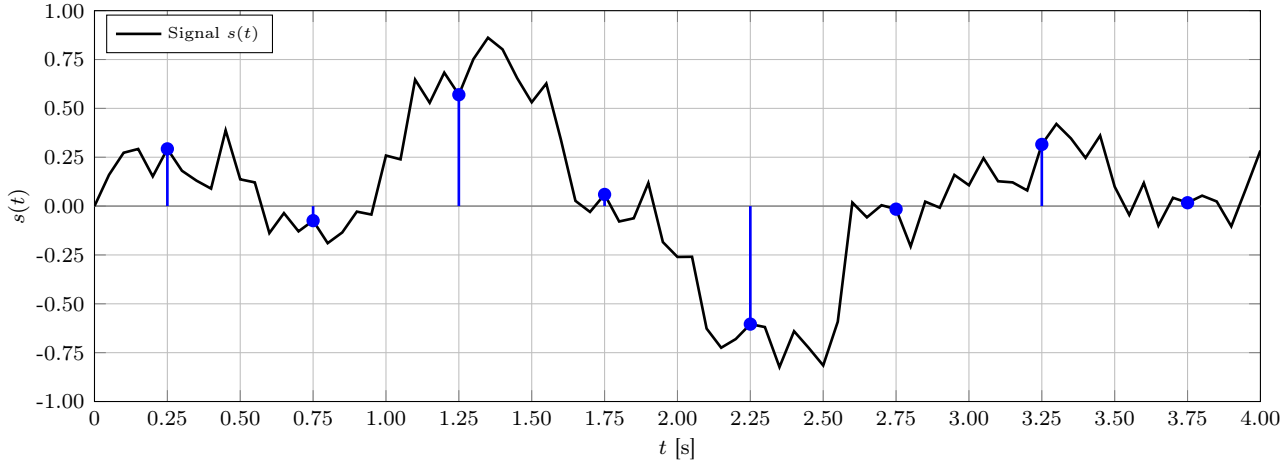
Abbildung 1.1: Zeit- und wertkontinuierliches Signal auf Empfängerseite
