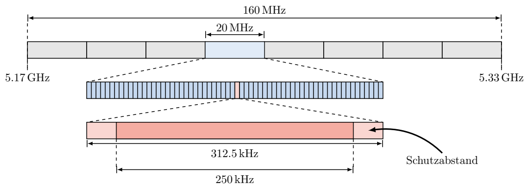
Abbildung 1: IEEE 802.11a Kanalaufteilung für Deutschland.
