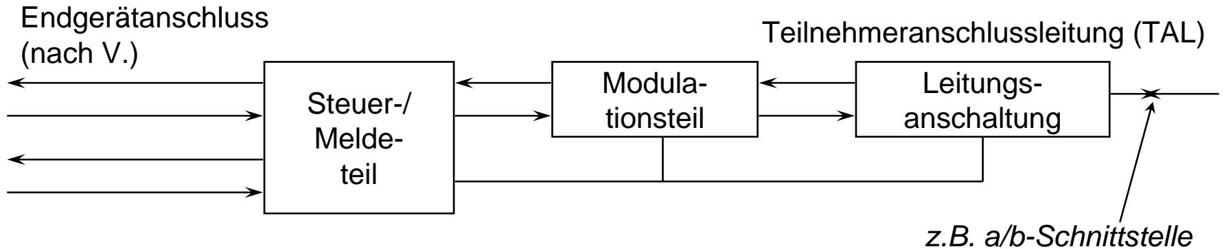
Schematischer Aufbau eines Modems
