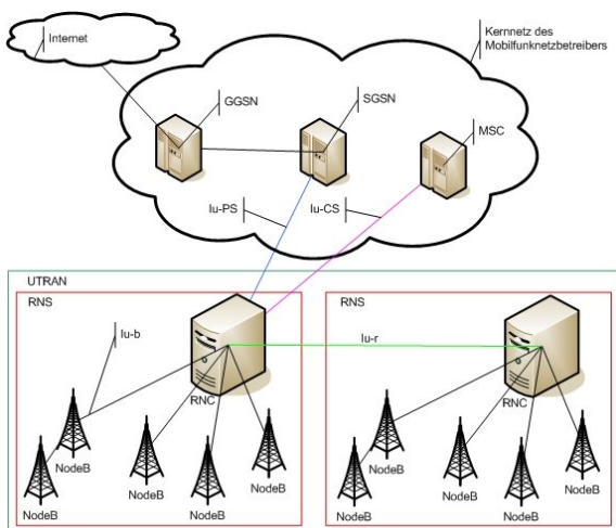
Abbildung 1: UMTS Netzstruktur
