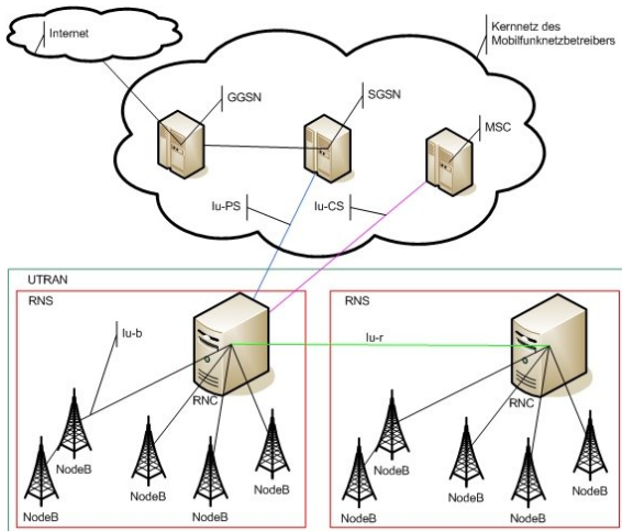
Abbildung 1: UMTS Netzstruktur
